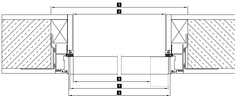
Coupe horizontale avec panneau de porte affleurant
