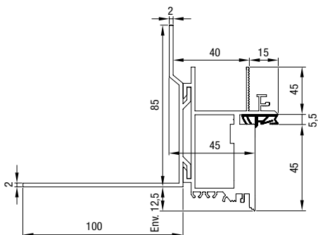
Dimensionnement huisserie Zeroline
